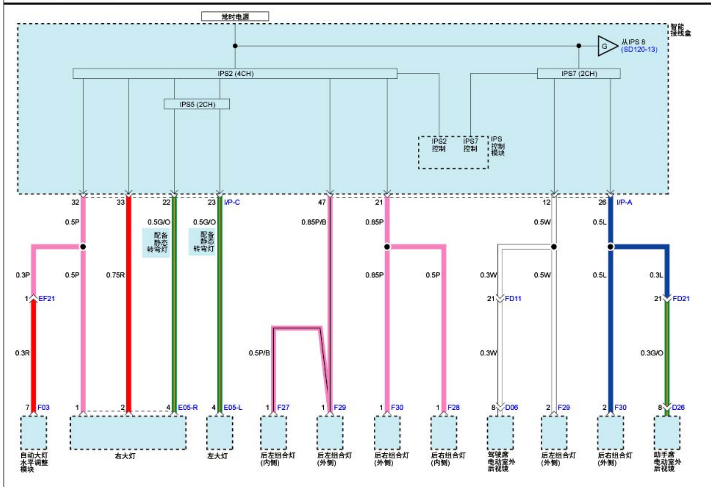
室内保险丝分布(12)
